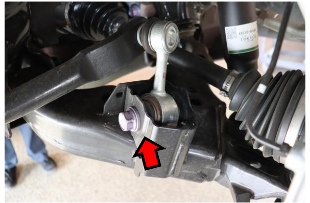
4. Remove the sway bar end link bolt.
